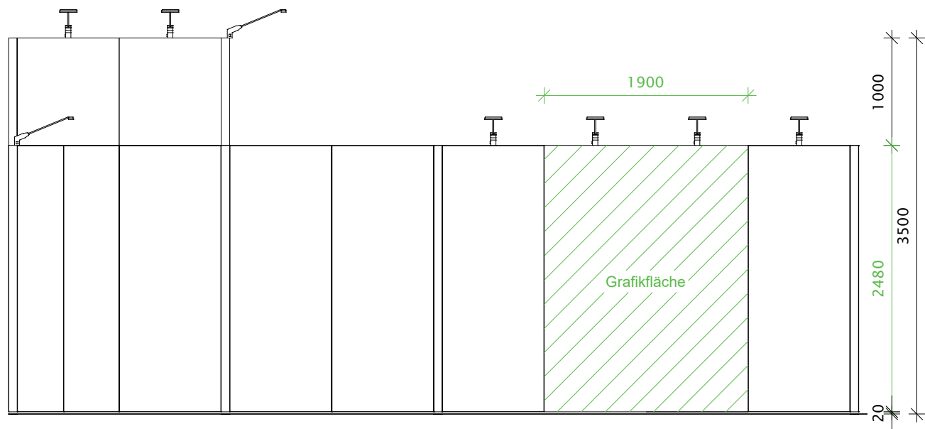
Frontansicht M 1:50,mm
