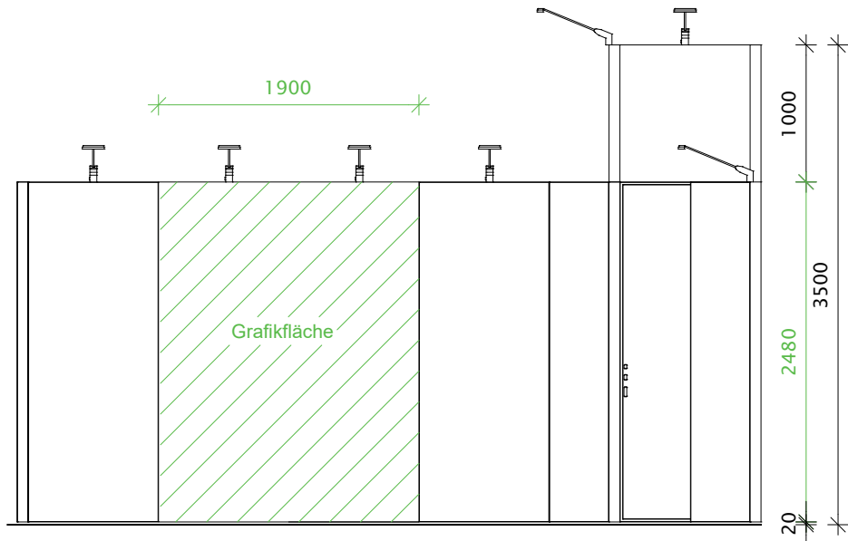
Seitenansicht rechst M 1:50,mm
