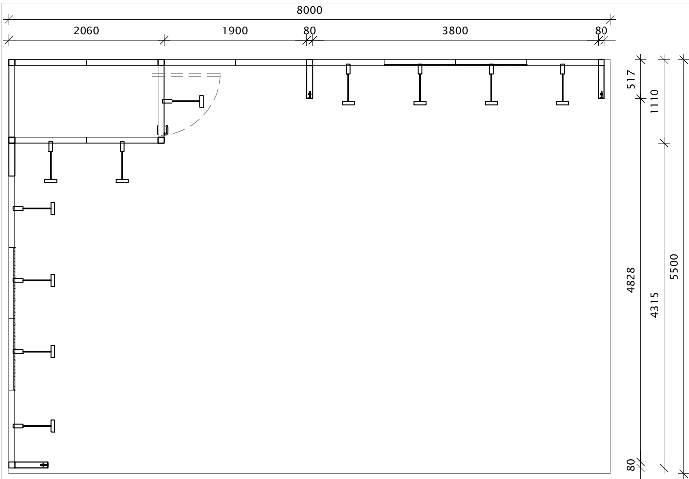
Grundriss M 1:50,mm
