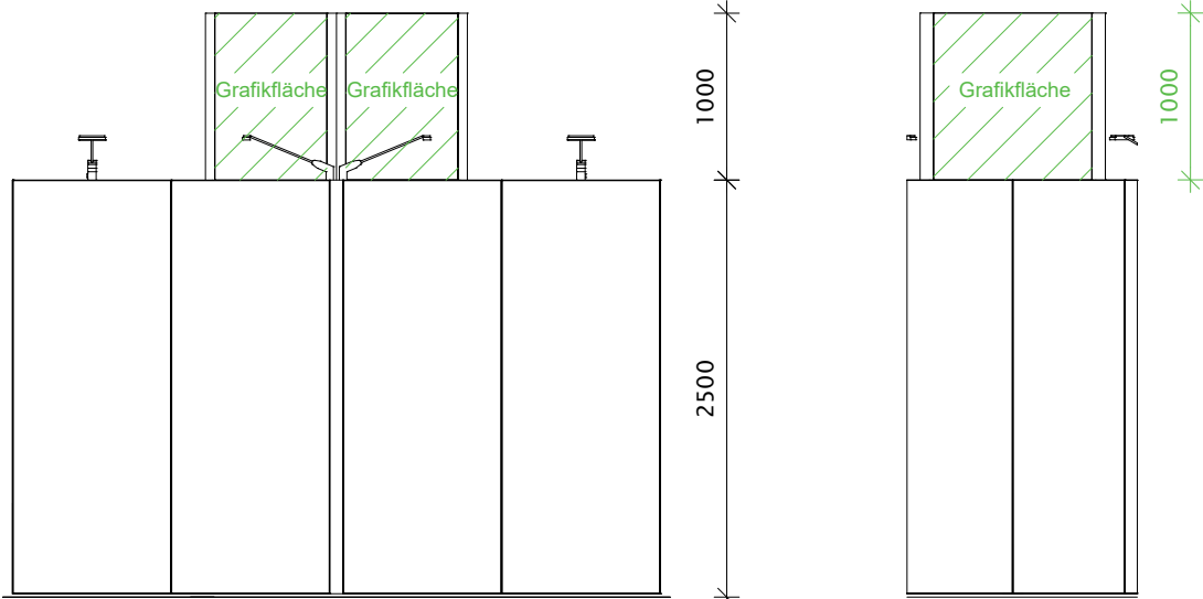
Seitenansicht rechst M 1:50,mm
