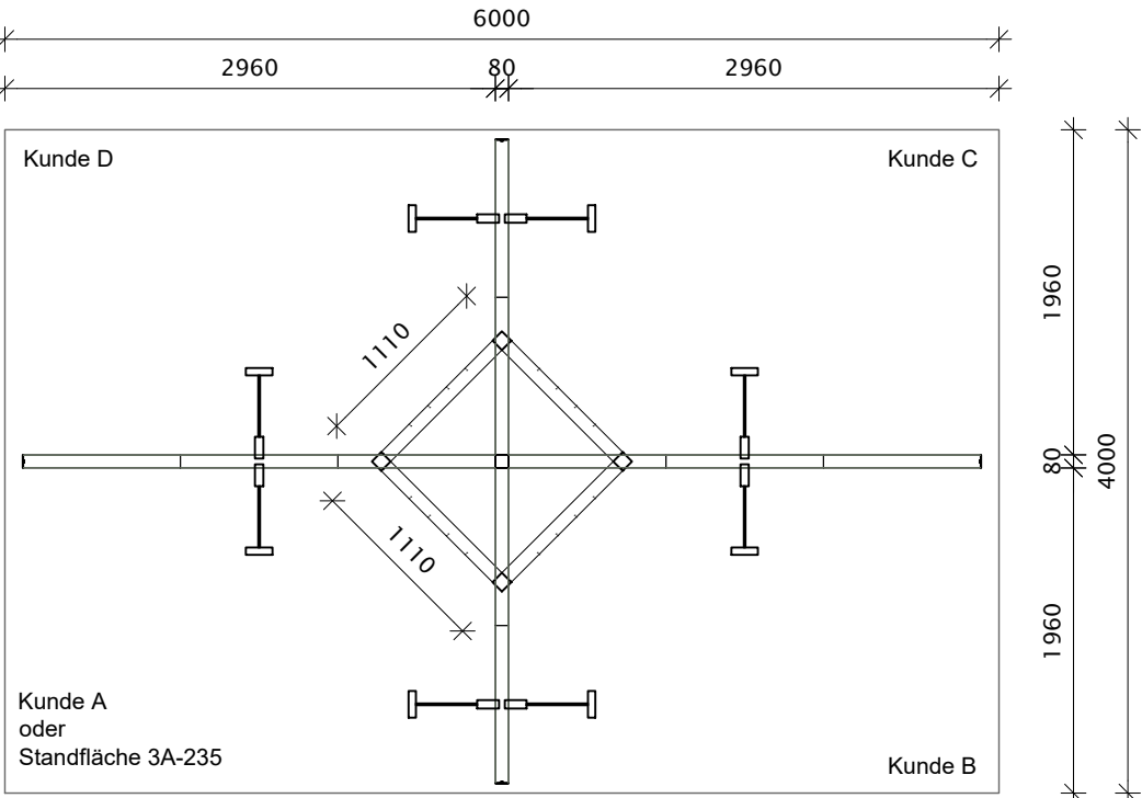
Grundriss M 1:50,mm
