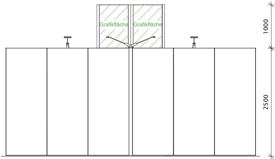
Frontansicht M 1:50,mm
