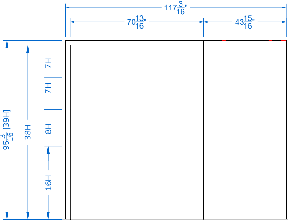
ELEVATION A
