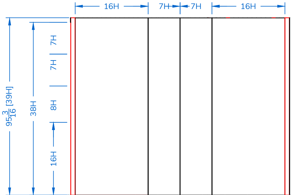
ELEVATION G
