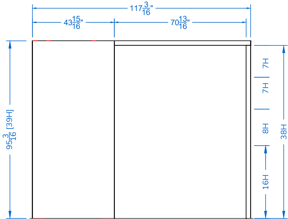
ELEVATION E
